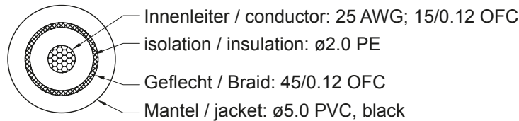
Querschnitt / Cross section
